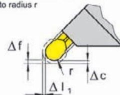
Korrektur-Faktoren \Delta l_1 , \Delta c und \Delta f im Verhältnis zum Radius r Revision factor \Delta l_1 , \Delta c and \Delta f in relation to radius r
