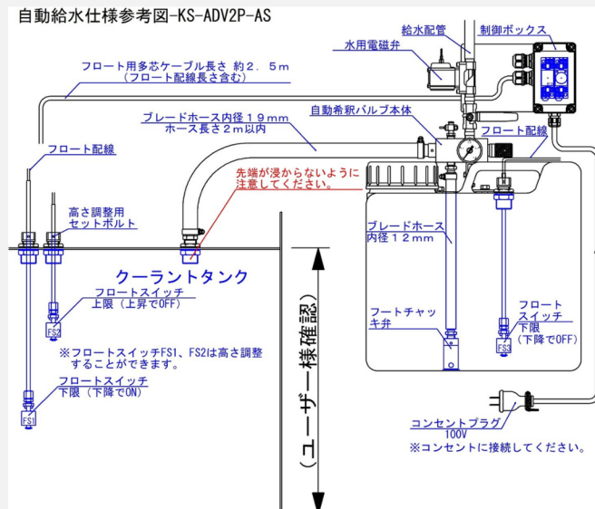
自動給水仕様参考図-KS-ADV2P-AS
