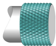
RGE 30° (DIN 82) Type B (ISO 13444)
